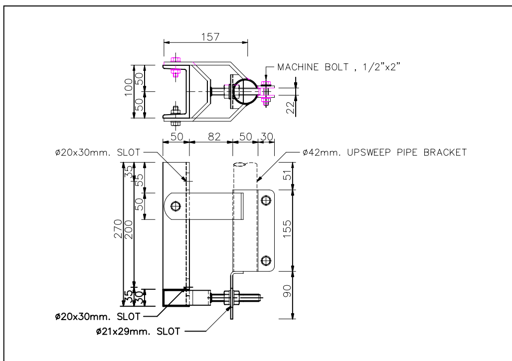
รูปที่ 1-4 แป้นติดกิ่งคอม (Bracket) อุปกรณ์ที่ติดกับเสาไฟฟ้า ผนัง หรือกำแพง เพื่อยึดกิ่งคอมไฟฟ้า และคอมไฟฟ้า
