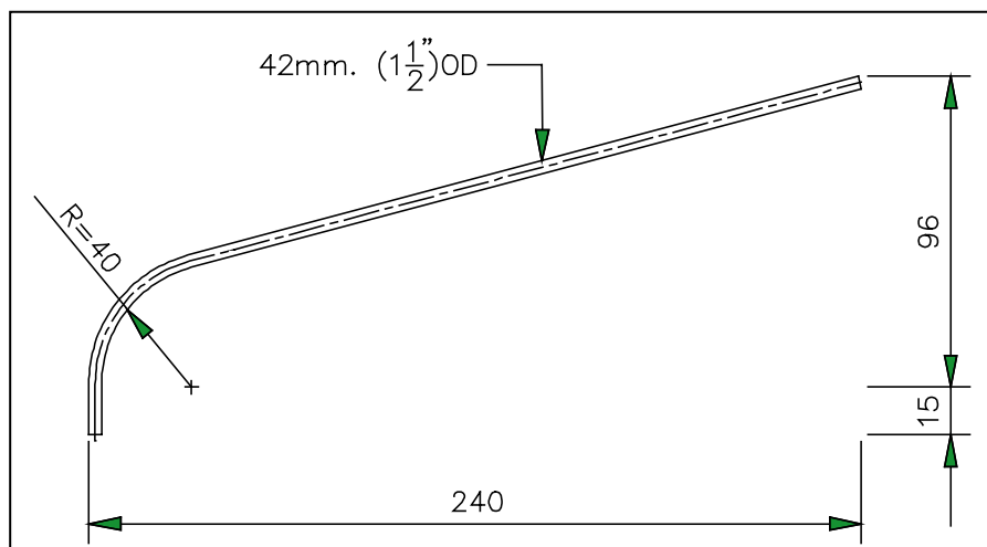
รูปที่ 1-3 กิ่งโคมไฟฟ้า (Rod หรือ Arm) อุปกรณ์ที่เชื่อมต่อกับโคมไฟฟ้า และแป้นกดกิ่งโคมเพื่อยื่นออกไปให้แสงสว่างแก่บริเวณที่ต้องการ
